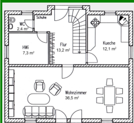
Grundriss Erdgeschoss 72qm
