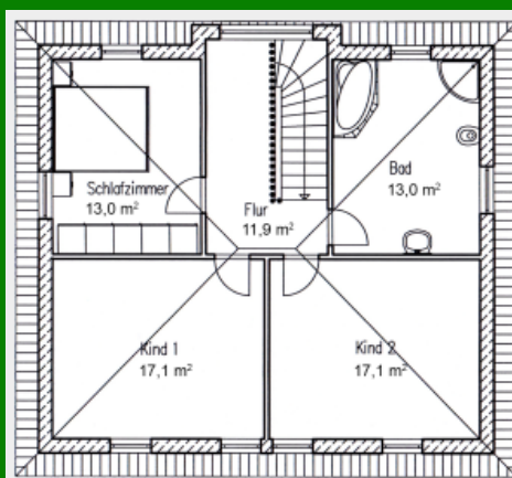
Grundriss Dachgeschoss 72qm
