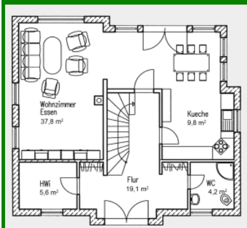
Ergeschoss 76,6qm
